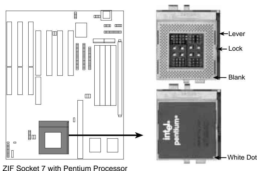
ZIF Socket 7 with Pentium Processor
